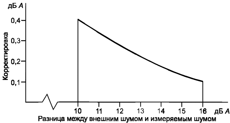
Рисунок 3.1а — Диаграмма корректировки уровня шума
