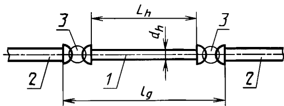
1 — высоковольтная проволока; 2 — подходящий провод длиной (120 \pm 2) мм; 3 — трубка
