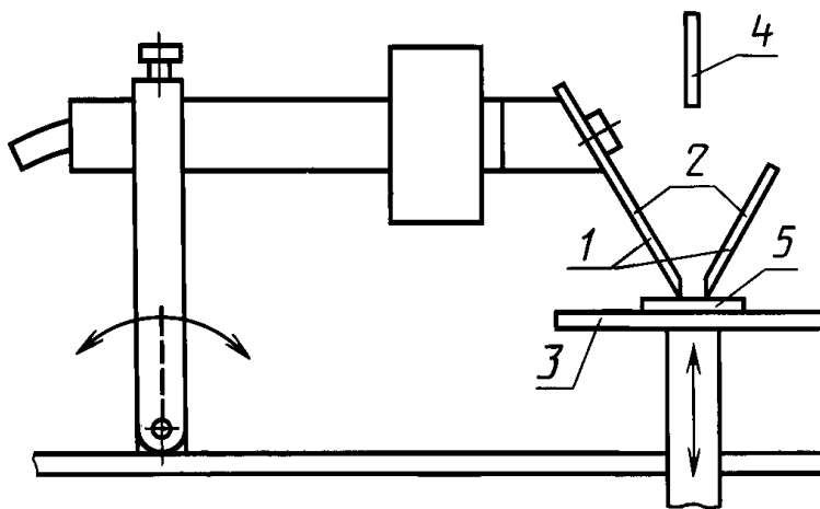
1 — электрод; 2 — медный удлинитель; 3 — опора; 4 — конец капельницы; 5 — образец
