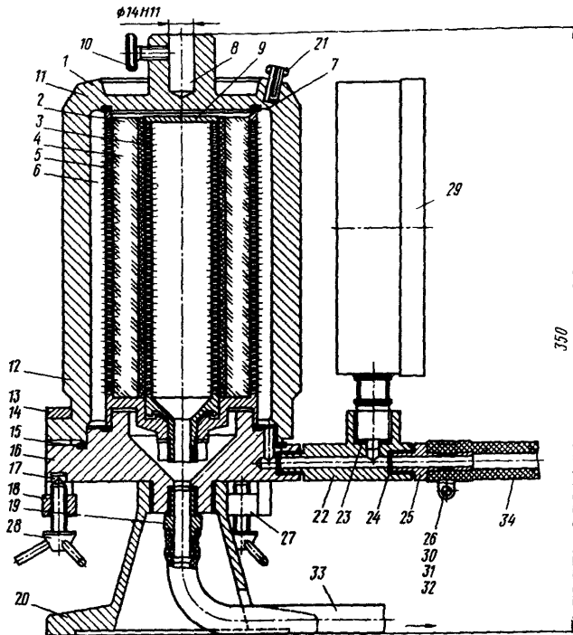
Рис.2. Схема прибора для определения кольматации геотекстиля: 1-корпус в сборе; 2-перфорированный цилиндр; 3-геотекстиль; 4-грунт; 5-форма; 6-кольцевой зазор; 7-отверстие; 8-гнездо; 9-заглушка; 10, 21, 28, 30-винты; 11, 12, 15, 23, 24, 27-прокладки; 13, 31-гайки; 14, 32-шайбы; 16-корпус; 17-вставка; 18, 26-хомуты; 19, 25-штуцера; 20-основание; 22-переходник; 29-манометр; 33-выходная трубка; 34-входная трубка
