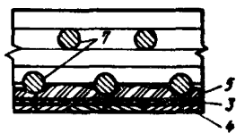
Рис.5. Устройство дренажа в конструкциях из буронабивных свай: 1-окно; 2-дренажная труба; 3-геотекстиль; 4-плиты; 5-грунт; 6-ростверк; 7-буронабивные сваи
