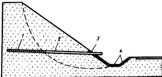
Рис.8. Примы- кание дрен к водоотводному лотку: 1-водо- приемная часть дрены; 2-водо- отводная часть дрены; 3-оголо- вок; 4-плитки
