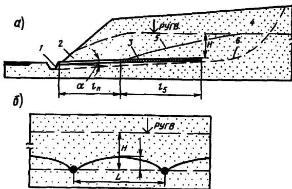
Рис.3. Схема бестраншейного горизонтального дренажа: 1-лоток; 2-водостводная часть дрены; 3-водоприемная часть дрены; 4-грунт; 5-уровень грунтовых вод после осушения грунтового массива; 6-поверхность скольжения
