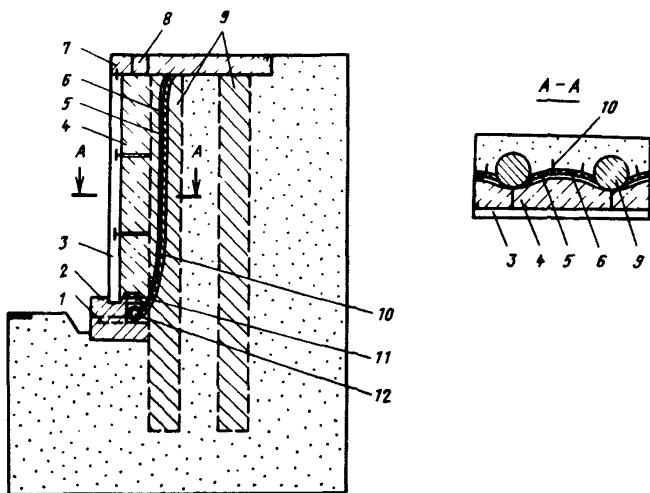
Рис.7. Застенный дренаж в конструкциях из буронабивных свай с монолитной облицовочной стенкой: 1-дренажное окно; 2-брус; 3-опалубка; 4-бетон; 5-пленка; 6-геотекстиль; 7-ростверк; 8-отверстие; 9-сваи; 10-штырь; 11-слой битума; 12-дренажная труба
