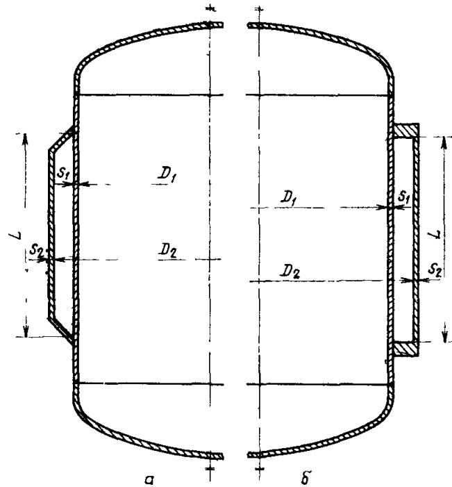
а—с сопряжением при помощи конуса; б—с сопряжением при помощи кольца
