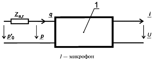
Рисунок 1 — Эквивалентная схема микрофона-приемника в свободном поле
