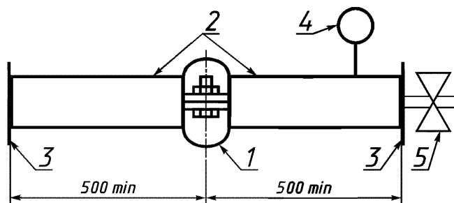
1 — муфта; 2 — трубопровод; 3 — заглушка; 4 — манометр (вакуумметр); 5 — запорное устройство
