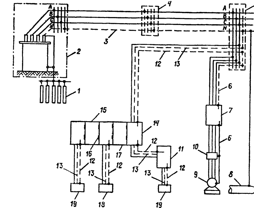
Рис. 3. Пример выполнения зануления в электроустановке системы автоматизации: 1 — заземлитель; 2 — понижающая трансформаторная подстанция автоматизируемого объекта; 3 — нулевой рабочий проводник, используемый в качестве магистрали зануления; 4 — промежуточный щит электроснабжения; 5 — распределительный щит электроснабжения, питающий систему автоматизации; 6 — нулевой рабочий проводник, который используется в качестве нулевого защитного проводника, зануляющего сборку питания задвижек, пускатель, электропривод; 7 — сборка питания задвижек; 8 — повторное зануление; 9 — электропривод задвижки; 10 — магнитный пускатель; 11 — местный щит контроля и управления; 12 — нулевой защитный проводник; 13 — нулевой рабочий проводник; 14 — панель питания системы автоматизации; 15 — щит контроля и управления в операторной; 16 — контактные металлические соединения панелей щита; 17 — рама щита; 18 — датчики, первичные приборы; 19 — отдельно стоящий прибор
