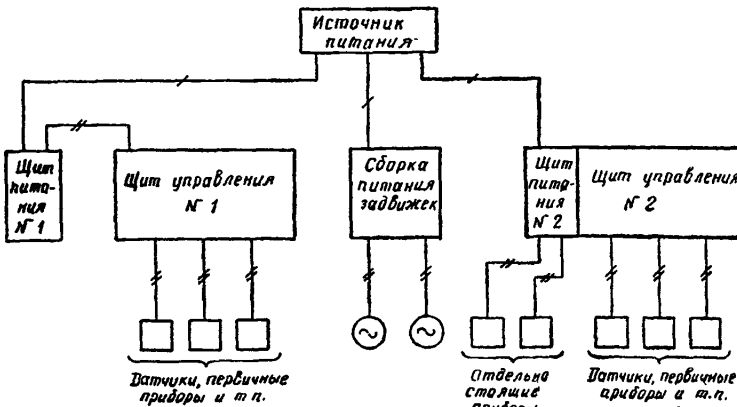
Рис. 1. Основные звенья схемы электропитания систем автоматизации (линия с одним штрихом — питающая сеть, с двумя штрихами — распределительная сеть)
