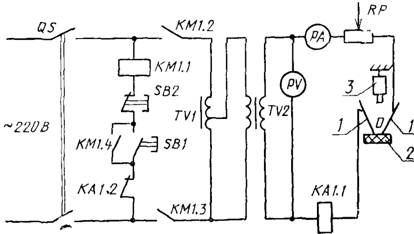
Принципиальная электрическая схема установки испытаний на трекингостойкость
