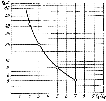
График определения минимального значения времени нагрева t_e
