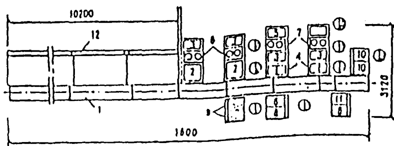
Рис. 10 Технологическое оборудование для отпуска комплексных обедов
