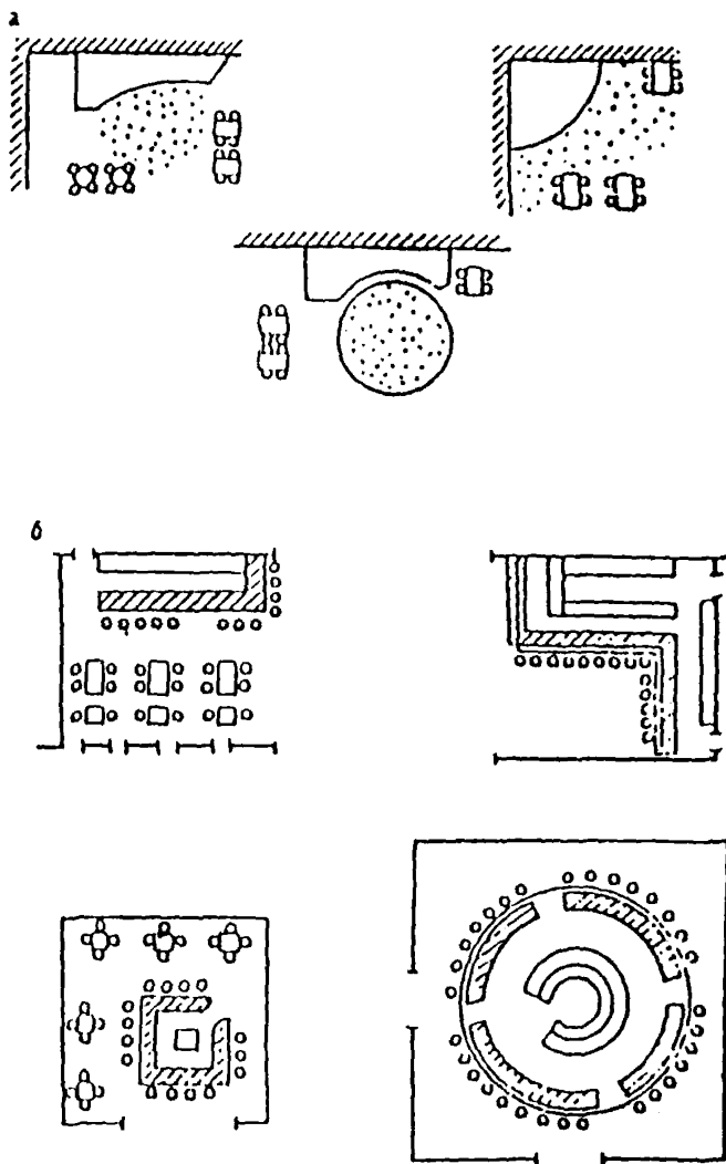
Рис. 12. Принципи розміщення і напозичіююше рішення зстрад, мест для таццв(а), барних стокк(б)
