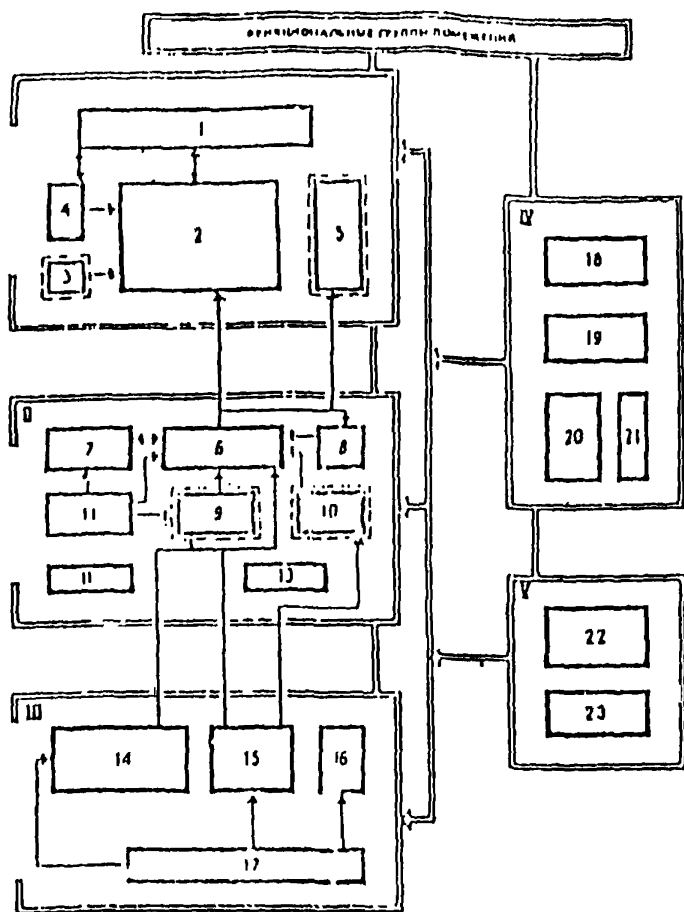
Рис. 1. Схемы взаимосвязи функциональных групп помещений логотобочных предприятий общественного питания с само- обслуживанием
