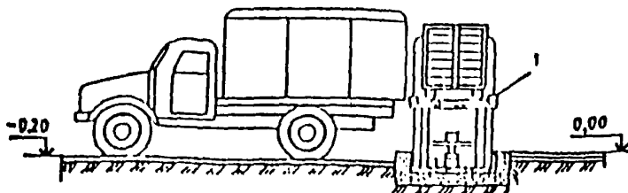
Рис. 13. Принципиальная схема организации погрузочно-разгрузочных работ в доготовочных предприятиях общественного питания
