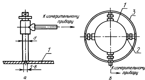
1 — стенка газохода; 2 — патрубок; 3 — соединительный трубопровод
