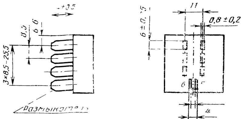
Вилка ВТ-6
