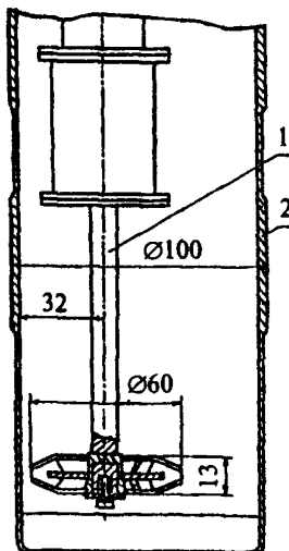
1 - лопастное устройство, 2 - стакан Рисунок 1 - Смеситель лопастной
