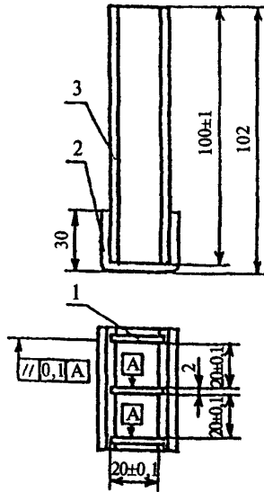
Рисунок 5 — Форма размером 20x20x100 мм
