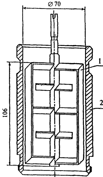
Рисунок 4 — Схема измерительного узла консистометра
