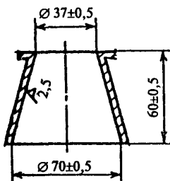
Рисунок 2 — Форма-конус
