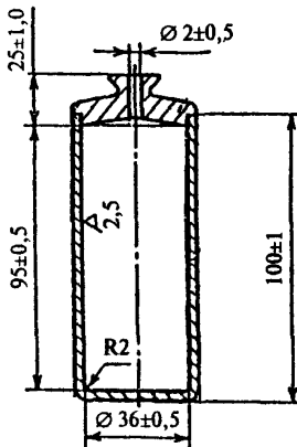
Рисунок 3 — Пикнометр
