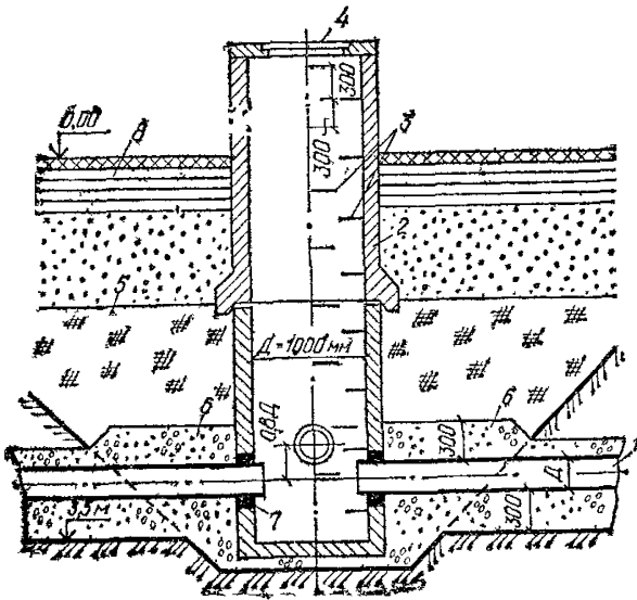
Рис. 21. Смотровой колодец (типовой проект Гипроводхоза)
