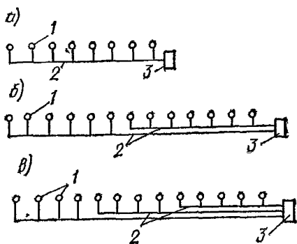
Рис. 88. Схемы линейных (тупиковых) сборных водоводов при линейном расположении водозаборных сооружений и концевом расположении сборного узла a — в одну нитку; б — в две нитки; в — в три нитки; 1 — водозаборы; 2 — сборные водоводы; 3 — сборный узел
