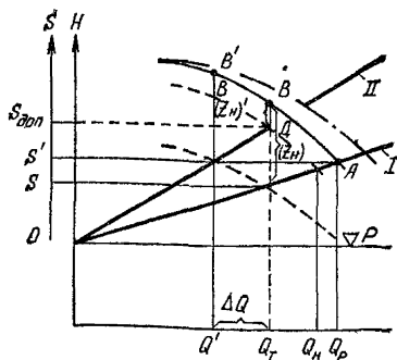
Рис. 101. Графоаналитический метод решения задачи регулирования производительности скважины
