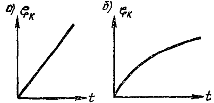
Рис. 59. Графики роста сопротивления скважин
