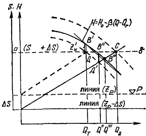
Рис. 102. Графоаналитический метод расчета прироста производительности скважины при ИППВ
