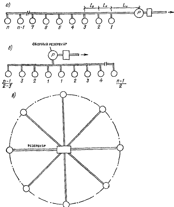
Рис. 96. Схемы подключения скважин к сборным водоводам
