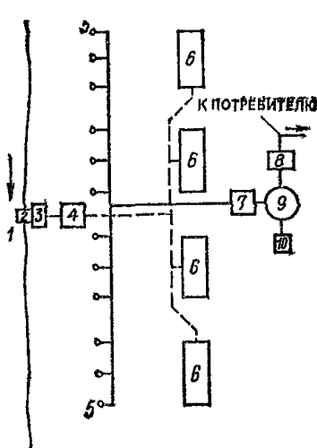
Рис. 46. Компонировочная схема СИП при однорядном расположении каптажных и инфильтрационных сооружений
