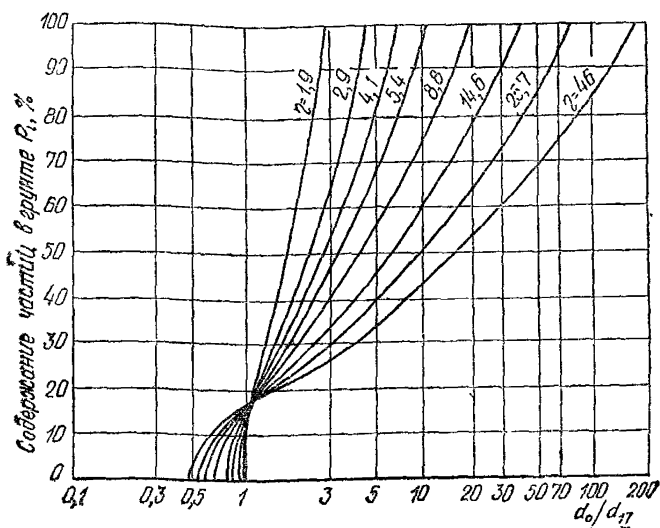
Рис. 32. Гранулометрический состав несuffозионных грунтов в относительных координатах
