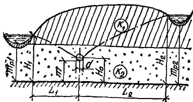
Рис. 26. Схема к расчету горизонтального водозабора в двухслойном водоносном пласте в междурусном массиве
