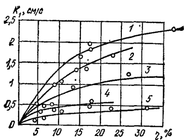
Рис. 10. Изменение проницаемости различных фильтров от скважности 1 — каркасно-стержневого; 2 — проволочного на трубчатом каркасе; 3 — с мостообразными отверстиями; 4 — с водоприемной поверхностью из штампованного листа; 5 — с сеткой галунного плетения
