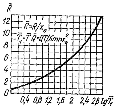
Рис. 70. График для определения протяженности ЗСО \bar{R} (к схеме рис. 69)
