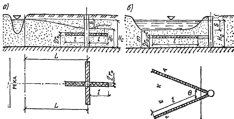
Рис. 42. Схемы к расчету производительности лучевых водозаборов а — береговой; б — подрусловый
