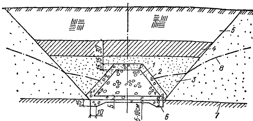
Рис. 15. Каменно-щебеночный водозабор
