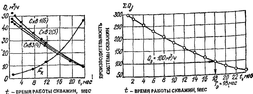
Рис. 107. Расчетные графики изменения во времени \zeta_h(t) , Q_j(t) и \Sigma Q(t) при действии скважин в режиме S_j = \text{const}
