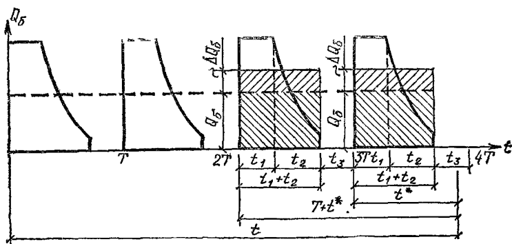
Рис. 60. Схема к расчету \Delta \tilde{h}
