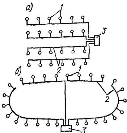
Рис. 88. Схемы линейных (тупиковых) сборных водоводов при линейном расположении водозаборных сооружений и концевом расположении сборного узла a — в одну нитку; б — в две нитки; в — в три нитки; 1 — водозаборы; 2 — сборные водоводы; 3 — сборный узел
