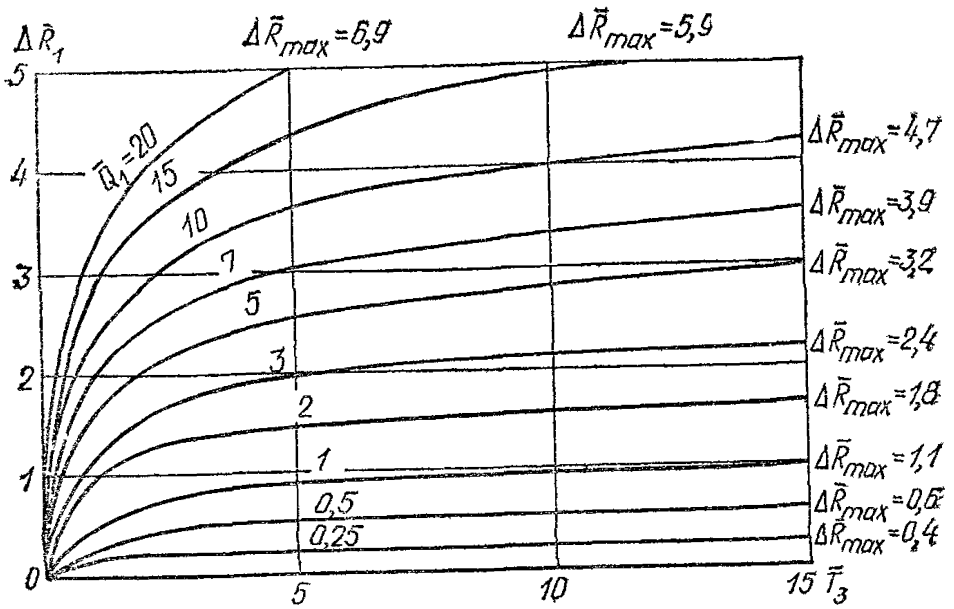
Рис. 78. График для определения протяженности ЗСО R (к схеме рис. 77, а) \Delta \bar{R}_1 = \Delta R / l + \bar{Q}_1 x_0 / l(1 + \bar{Q}_1) ; \bar{T}_3 = \Gamma q / mn l + x_0 / l(1 + \bar{Q}_1) ; \Delta \bar{R}_{max} = \Delta R_{max} / x_0 ; \bar{Q}_1 = \bar{Q} / \bar{l}^2 = Q x_0 / \pi q l^2 ; \bar{l} = l / x_0
