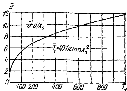
Рис. 71. График для определения ширины ЗСО \bar{d} (к схеме рис. 69)
