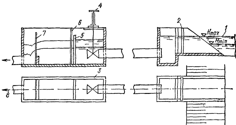
Рис. 51. Схема входного узла с водосливом
