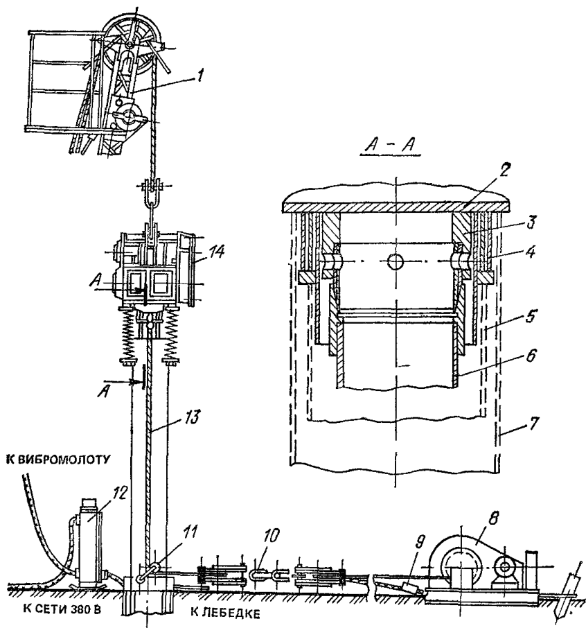
Рис. 3. Вибромолот БВС-1 для погружения и извлечения обсадных труб при ударно-канатном бурении скважин на воду
