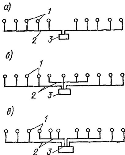
Рис. 89. Схемы линейных (тупиковых) сборных водоводов при линейном расположении водозаборных сооружений и центральном расположении сборного узла a — в две нитки; б — в три нитки; в — в четыре нитки 1 — водозаборы; 2 — сборные водоводы; 3 — сборный узел
