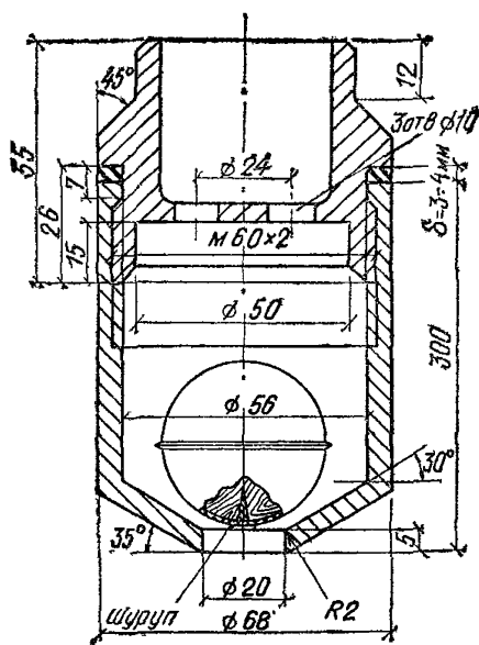
Рис. 118. Коническое седло с плавающим шаровым клапаном и перфорированной перегородкой
