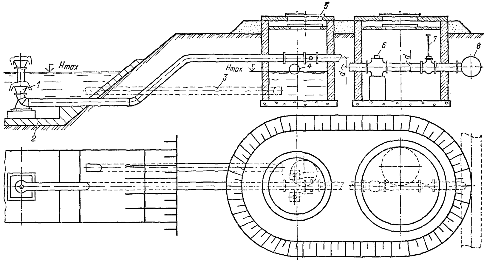
Рис. 50. Схема входного узла (закрытая распределительная сеть)
