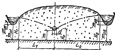
Рис. 25. Схема к расчету горизонтального водозабора в однослойном водоносном пласте в междурусном массиве
