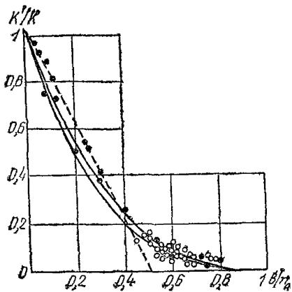
Рис. 59. Графики роста сопротивления скважин
