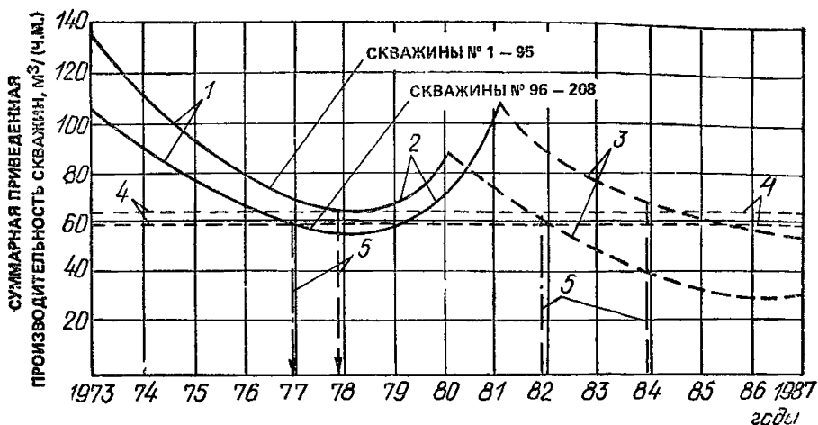
Рис. 114. Изменение во времени суммарной удельной производительности самозливающихся скважин дренажной системы
