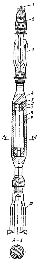
Рис. 2. Виброударный буровой снаряд ВС для ударно-канатных станков
