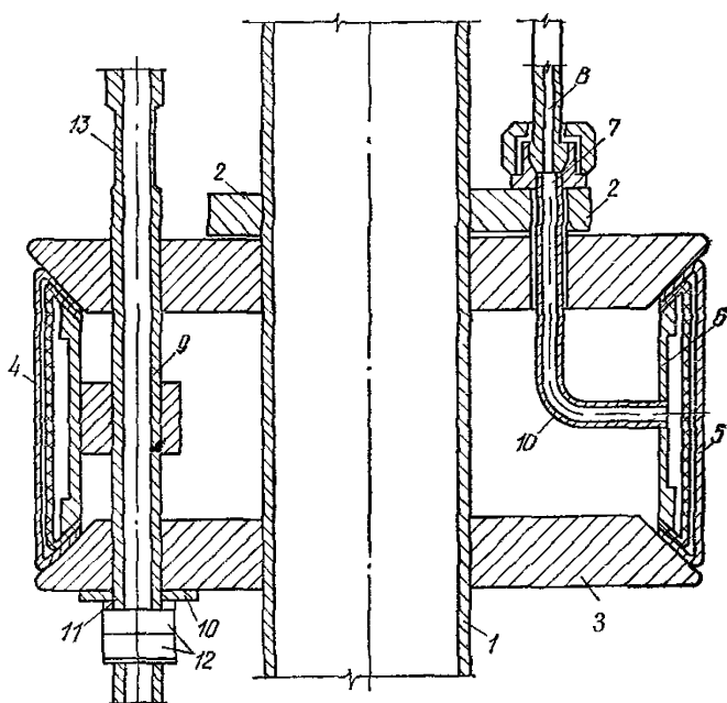
Рис. 111. Пневматический пакер
