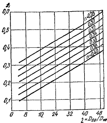
Рис. 34. График j_* = f_*(\eta)
