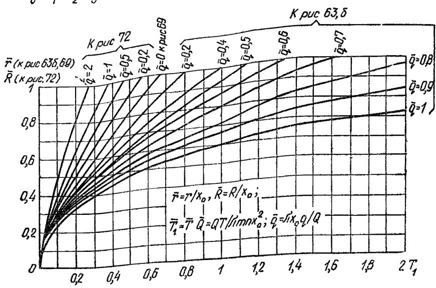
Рис. 66. График для определения протяженности ЗСО r (к схемам рис. 63, б, 69) и R (к схеме рис. 72)
