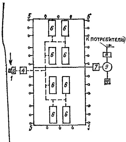
Рис. 47. Компонировочная схема СИП при двухрядном расположении бассейнов и контурном размещении скважин
