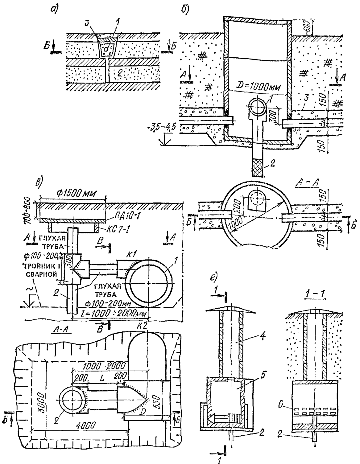
Рис. 20. Комбинированный горизонтальный водозабор с вертикальными скважинами-усилителями
