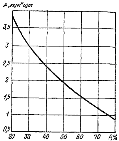
Рис. 54. График зависимости обобщенного параметра A = K \gamma_{ск} от процентного (по весу) содержания в воде, подаваемой на инфильтрацию, мелкопылеватых и глинистых фракций P
