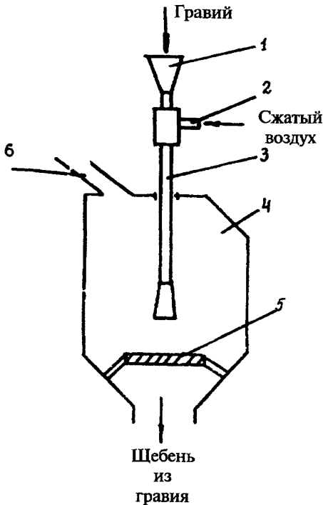
Схема пневмоударной дробилки:
