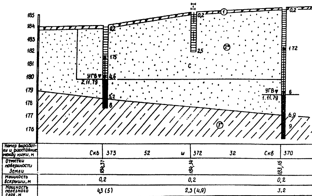
Геолого-литологический разрез 11
