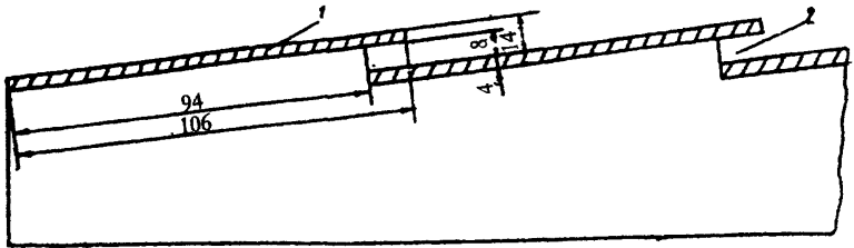
Рис. 3. Уступообразное днище:
