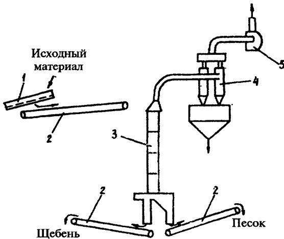
Рис. 4. Схема технологической линии ВНИИнефуда для переработки отсеков дробления «сухим» способом:
