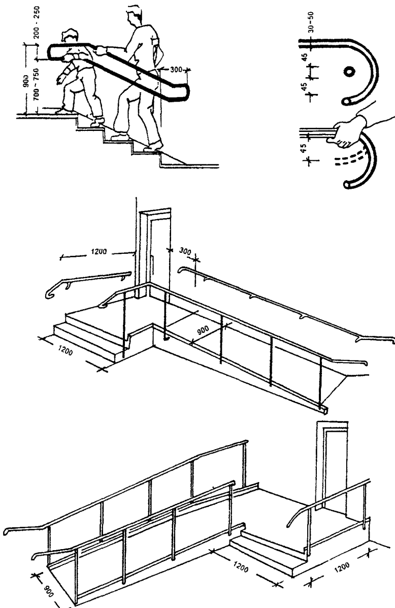
РИС 38 ПРИМЕРЫ УСТРОЙСТВА ВХОДНЫХ ЛЕСТНИЦ И ПАНДУСОВ
