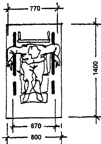
РИС 35 ГАБАРИТЫ КОЛЯСОК, ПРИМЕНЯЕМЫХ ДЛЯ ПЕРЕДВИЖЕНИЯ ИНВАЛИДОВ-ОПОРНИКОВ
