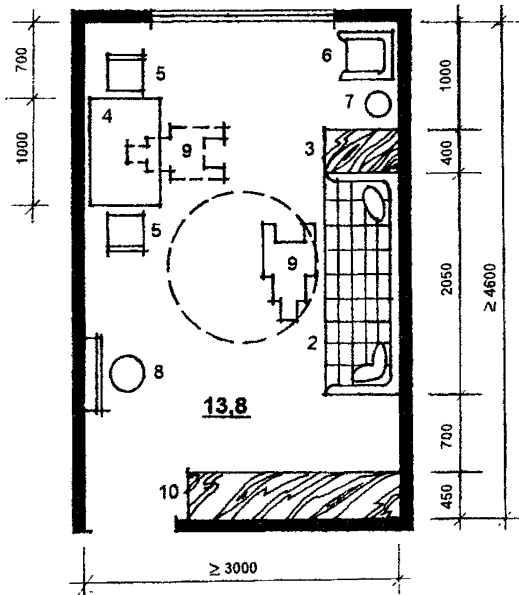
РИС.4.1. ПЛАНИРОВОЧНЫЕ СХЕМЫ ОДНОМЕСТНОЙ СПАЛЬНОЙ КОМНАТЫ
