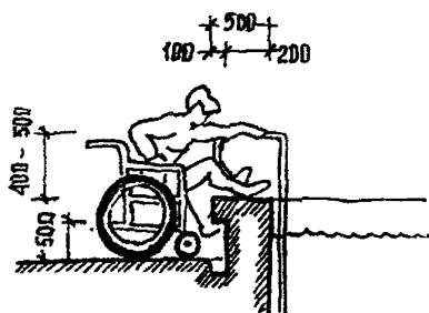
2а - без пандуса
