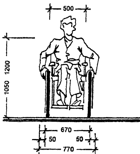
РИС 35 ГАБАРИТЫ КОЛЯСОК, ПРИМЕНЯЕМЫХ ДЛЯ ПЕРЕДВИЖЕНИЯ ИНВАЛИДОВ-ОПОРНИКОВ
