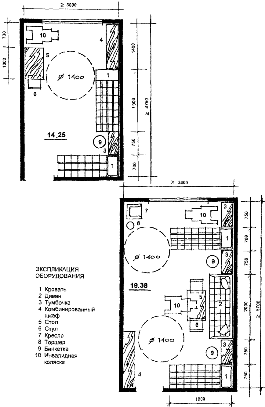
РИС 4.2 ПЛАНИРОВОЧНЫЕ СХЕМЫ СПАЛЬНЫХ КОМНАТ НА 2 И 3 МЕСТА
