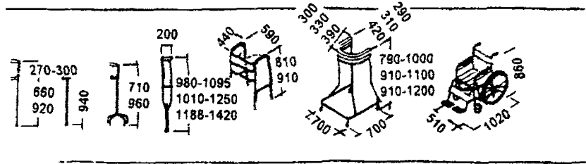
РИС.3.4 НЕОБХОДИМЫЕ ГАБАРИТЫ КОММУНИКАЦИЙ, УСТРОЙСТВ И СРЕДСТВ ПЕРЕДВИЖЕНИЯ ИНВАЛИДОВ
