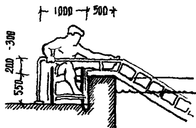
2б - с пандусом
