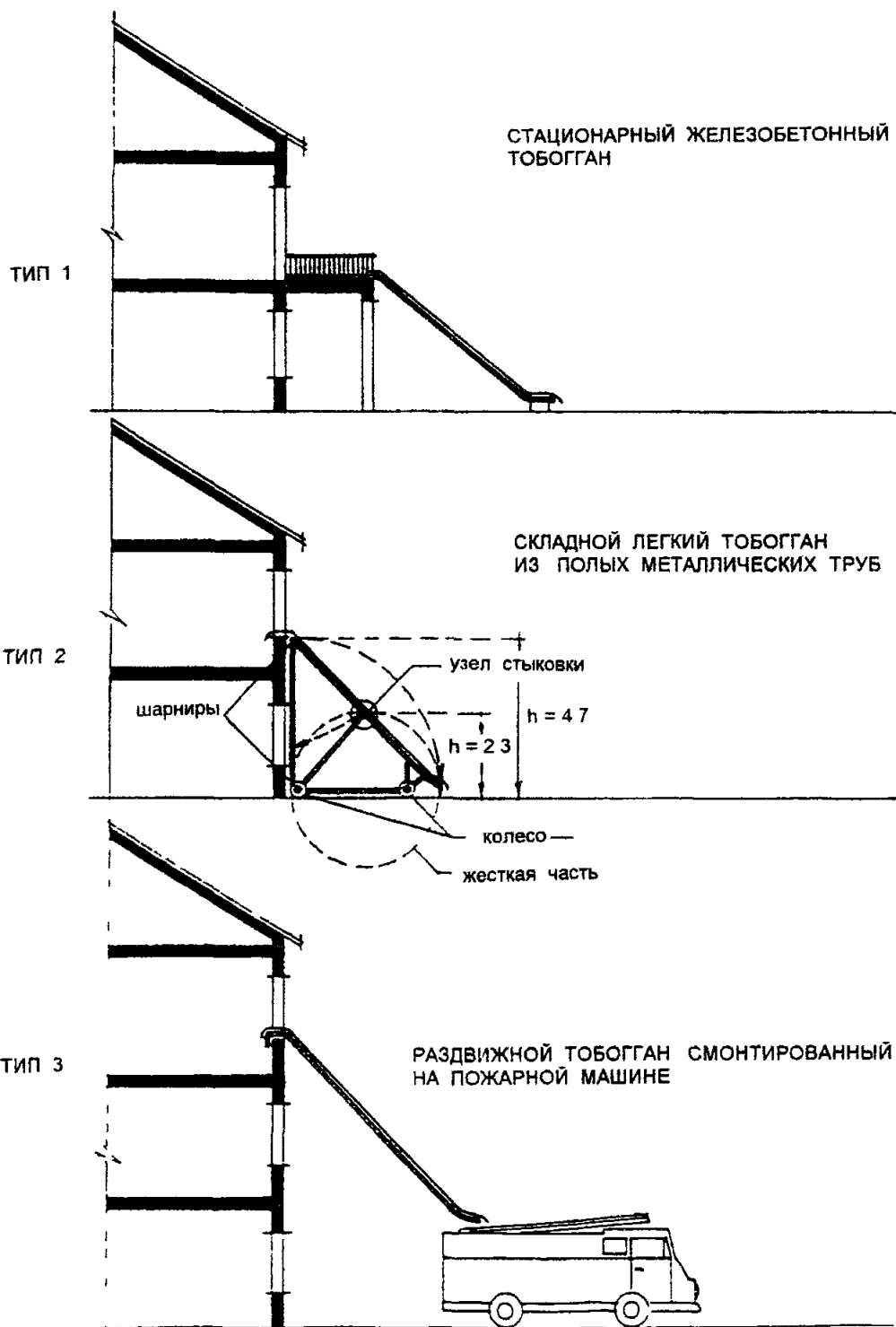
РИС 3 10 СХЕМЫ ТОБОГАНОВ
