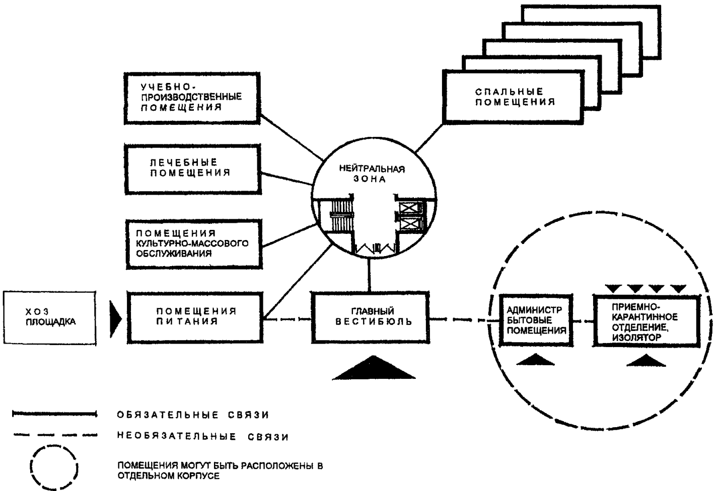
РИС 3 1 СХЕМА ФУНКЦИОНАЛЬНОЙ ВЗАИМОСВЯЗИ ОТДЕЛЬНЫХ ГРУПП ПОМЕЩЕНИЙ ДОМА-ИНТЕРНАТА ДЛЯ ПРЕСТАРЕЛЫХ И ИНВАЛИДОВ
