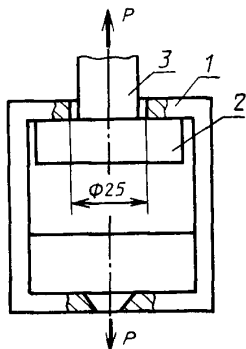
1—захват образца, 2—образец, 3—металлический цилиндр,
