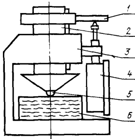
1—пластина; 2—пуансон; 3—корпус; 4—индикатор; 5—шарик; 6—образец
