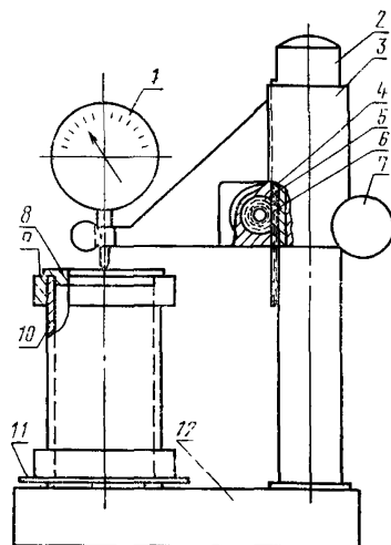
Прибор ГОИ
