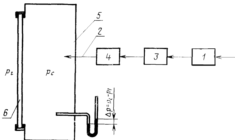
1—вентилятор (компрессор), 2—трубопровод; 3—регулятор потока воздуха; 4—измерительный прибор для измерения количества воздуха, 5—камера для создания избыточного давления, 6—испытываемый образец, P_i —давление воздуха на внутренней поверхности образца, P_c —давление воздуха на внешней поверхности образца
