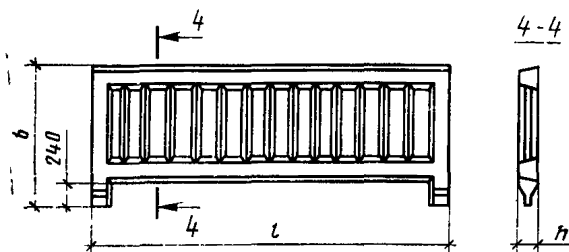
Панель ограждения платформы
