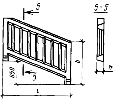
Панель ограждения лестничного марша
