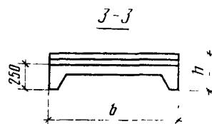
Панель ограждения лестничного марша
