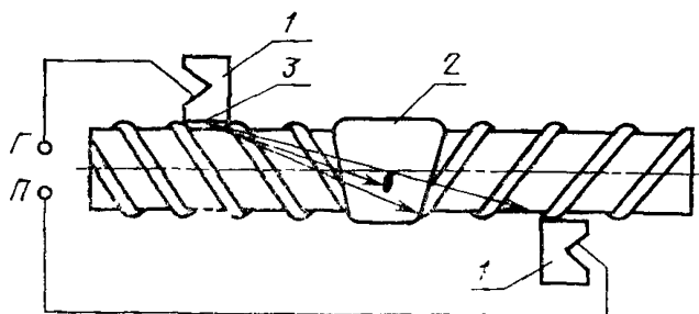
1—наклонные искатели; 2—сварное соединение; 3—метка, соответствующая точке выхода луча (ГОСТ 14782—76); Γ — вывод к генератору ультразвуковых колебаний; П — вывод к приемнику.
