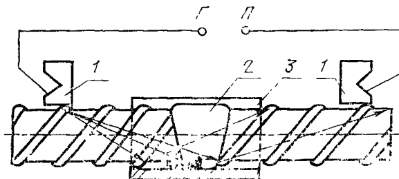
1—наклонные искатели; 2—сварное соединение; 3—скоба-накладка; Γ—вывод к генератору ультразвуковых колебаний; П—вывод к приемнику.
