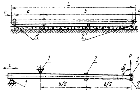
Схема испытания стоек
