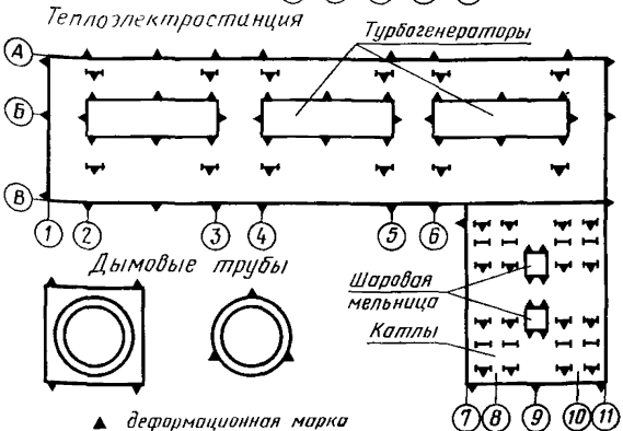
▲ деформационная марка
