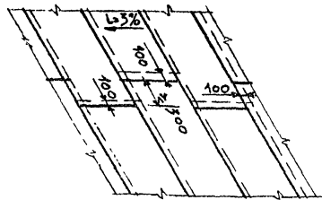
РАСКЛАДКА РУЛОННЫХ МАТЕРИАЛОВ ПРИ ТРЕХСЛОЙНОМ КРОВЕЛЬНОМ КОВРЕ
