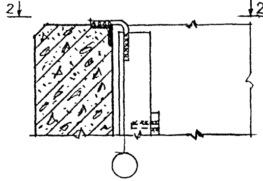
КРЕПЛЕНИЕ ПАНЕЛЕЙ В УГЛУ ПРИ ПРИВЯЗКЕ „250“
