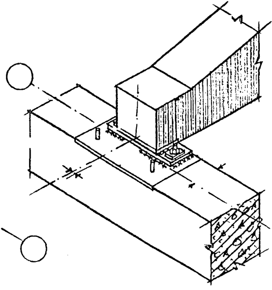
ОПИРАНИЕ СТРОПЬЯНОЙ ФЕРМЫ В СЕРЕДИНЕ ПРО- ЛЕТА ПОДСТРОПЬЯНОЙ ФЕРМЫ
