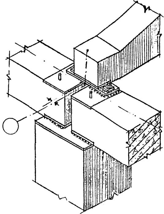
ОПИРАНИЕ ПОДСТРОПЬЯНЫХ ФЕРМ НА КОЛОННУ И СТРОПЬЯН- НОЙ ФЕРМЫ НА ПОДСТРОПЬЯНЫЕ
