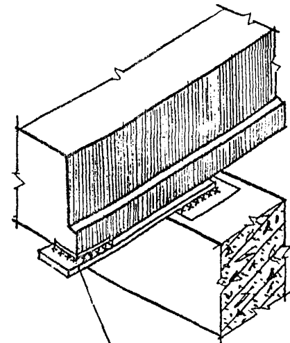
ОПИРАНИЕ ПЛИТ НА ФЕР- МЫ У ТОРЦОВ И ТЕМПЕРА- ТУРНЫХ ШВОВ ЗДАНИЯ
