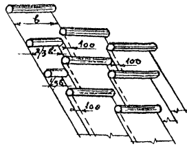
РАСКЛАДКА РУЛОННЫХ МАТЕРИАЛОВ ПРИ ТРЕХСЛОЙНОМ КРОВЕЛЬНОМ КОВРЕ
