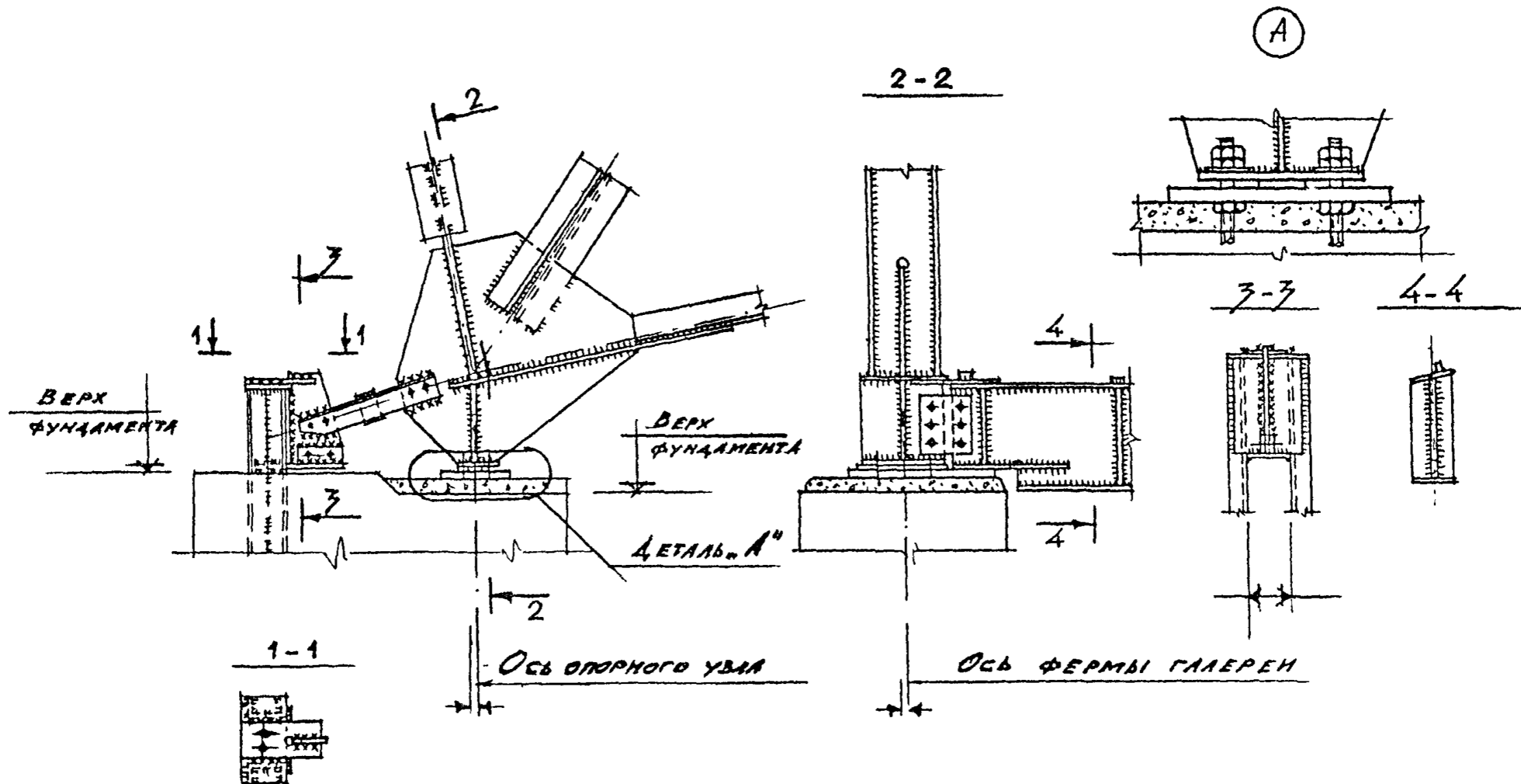
СХЕМА УЗЛА ФЕРМЫ ТРАНСПОР- ТЕРНОЙ ГАЛЕРЕИ
