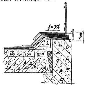
ДЕТАЛЬ УСТАНОВКИ ВОДОСТОЧНОЙ ВОРОНКИ
