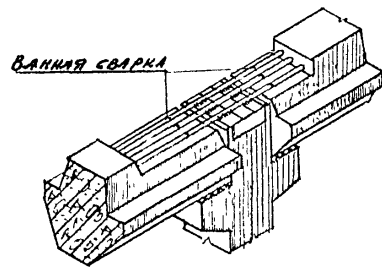
СХЕМА УЗЛОВ СОПРЯЖЕНИЯ РИГЕЛЕЙ С КРАЙНЕЙ И СРЕДНЕЙ КОЛОННАМИ В ВЕРХНЕМ ЭТАЖЕ, У ТОРЦОВ ЗДАНИЯ И ТЕМПЕРАТУРНЫХ ШВОВ
