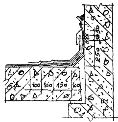
ДЕФОРМАЦИОННЫЙ ШОВ С ГИБКИМ КОМПЕНСАТОРОМ
