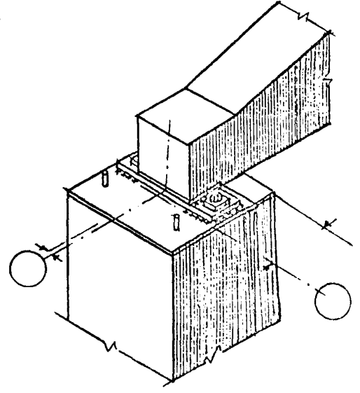
КРЕПЛЕНИЕ СТРОПЬЯН- НОЙ ФЕРМЫ К КОЛОННЕ СРЕДНЕГО РЯДА
