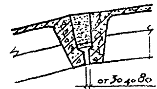
ЗАДЕЛКА ШВОВ МЕЖДУ ПЛИТАМИ У ПЕРЕЛОМОВ ВЕРХНЕГО ПОЯСА СТРОПНАБНЫХ ФЕРМ И БАЛОК
