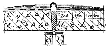
ДЕФОРМАЦИОННЫЙ ШОВ С ГИБКИМ КОМПЕНСАТОРОМ
