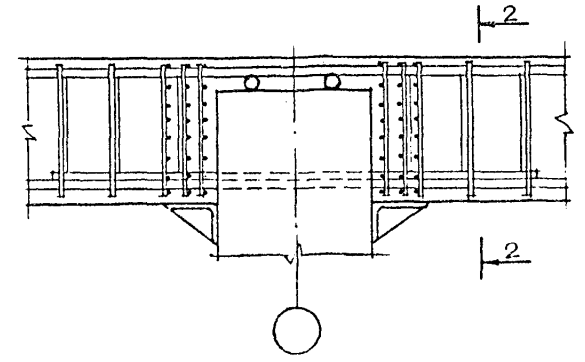
УЗЕЛ КРАЙНЕГО МОНОЛИТНОГО РИГЕЛЯ ПО СРЕДНИМ РЯДАМ КОЛОНН В УРОВНЕ ПОКРЫТИЯ
