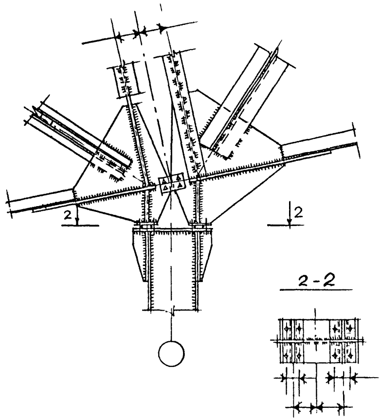
СХЕМЫ УЗЛОВ КОНСТРУКЦИИ ТРАНСПОРТЕРНЫХ ГАЛЕРЕЙ
