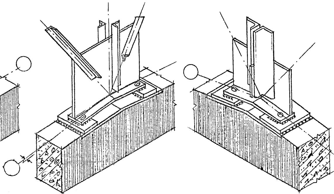
КРЕПЛЕНИЕ СРЕДНИХ СТОЕК ФЕРМ ФОНАРЯ
