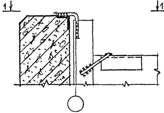
КРЕПЛЕНИЕ ПАНЕЛЕЙ В УГЛУ ПРИ ПРИВЯЗКЕ „0“
