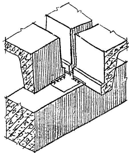
СТАЛЬНОЙ ЭЛЕМЕНТ ПРИВА- РЕНТЪ КЪ ФЕРМЕ ДО УСТА - НОВКИ ПЛИТЫ ПОКРЫТИЯ
