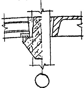
КРЕПЛЕНИЕ МЕЖКОЛООННЫХ ПЛИТ ПЕРЕКРЫТИЯ К РИГЕЛЯМ У СРЕДНЕЙ КОЛОНЫ
