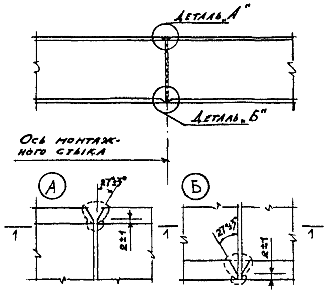
СХЕМА 25А
