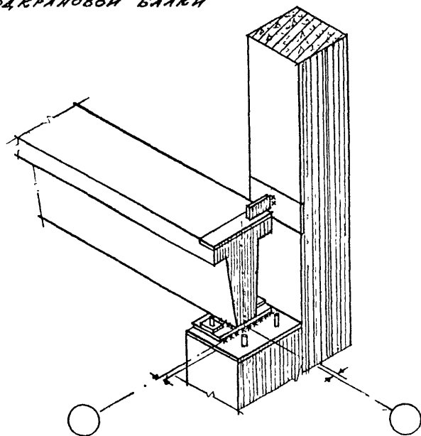
КРЕПЛЕНИЕ ЖЕЛЕЗОБЕТОННОЙ ПОДКРАНОВОЙ БАЛКИ
