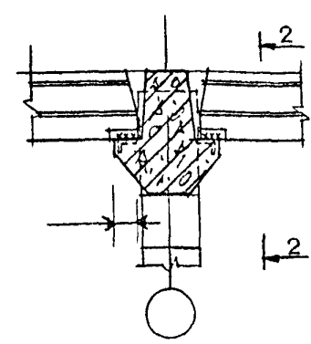
СХЕМА УЗЛОВ КРЕПЛЕНИЯ ПЛИТ ПЕРЕКРЫТИЯ И СОПРЯЖЕНИЯ МЕЖКОЛООННЫХ ПЛИТ ПЕРЕКРЫТИЯ И ПЕРЕКРЫТИЯ
