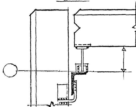
СХЕМА УЗЛОВ КРЕПЛЕНИЯ СТЕНОВЫХ ПАНЕЛЕЙ ПАРАПЕТА К НАСАДКЕ ФАХВЕРКА
