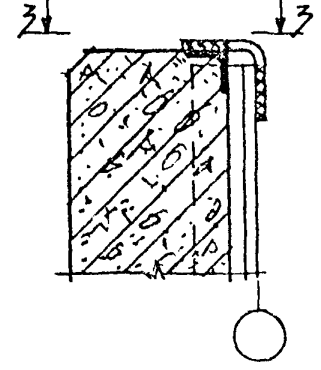
КРЕПЛЕНИЕ ПАНЕЛЕЙ СРЕДНЕГО РЯДА
