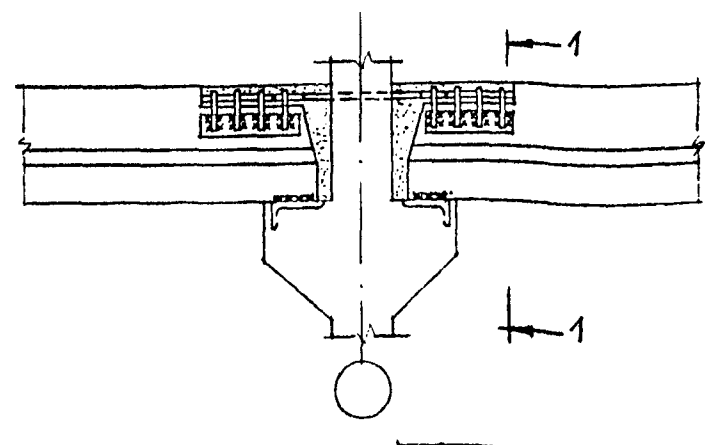
СХЕМА СОПРЯЖЕНИЯ РИГЕЛЕЙ С КОЛОННАМИ С ВАМОНОЛИНОВАНИЕМ УЗЛОВ БЕТОНОМ. СЕРИИ МН20/70 И 1.420-12
