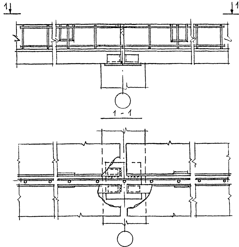
СХЕМА СОПРЯЖЕНИЯ ПАНТ ПОКРЫТИЯ СО СТОПНАВНЫМИ КОНСТРУКЦИЯМИ
