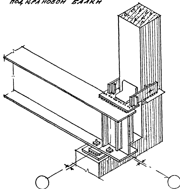
КРЕПЛЕНИЕ СТАЛЬНОЙ ПОДКРАНОВОЙ БАЛКИ
