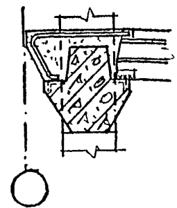
КРЕПЛЕНИЕ МЕЖКОЛООННЫХ ПЛИТ ПЕРЕКРЫТИЯ К РИГЕЛЯМ У СРЕДНЕЙ КОЛОНЫ
