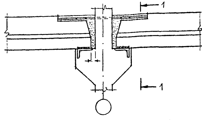
СОПРЯЖЕНИЕ РИГЕЛЕЙ СО СРЕДНЕЙ КОЛОННОЙ У ТОРЦОВ И ТЕМПЕРАТУРНЫХ ШВОВ ЗДАНИЯ
