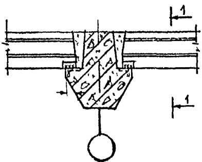
КРЕПЛЕНИЕ РЯДОВЫХ ПЛИТ ПЕРЕКРЫТИЯ И ПЕРЕКРЫТИЯ К РИГЕЛЯМ РЯДОВЫХ РАМ
