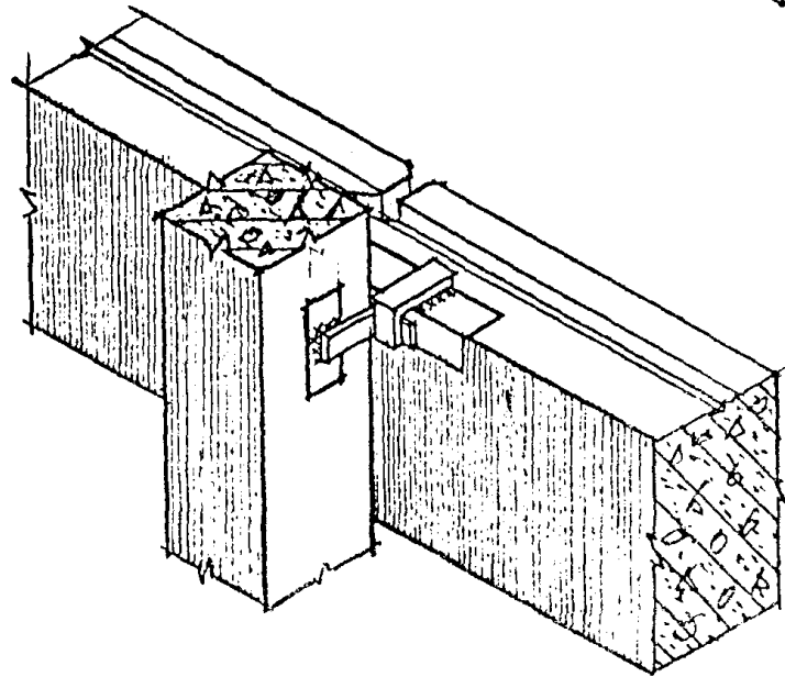
СХЕМА УЗЛОВ ХРЕПЛЕНИЯ ПАНЕЛЕЙ СТЕНОВОГО ОГРАЖДЕНИЯ
