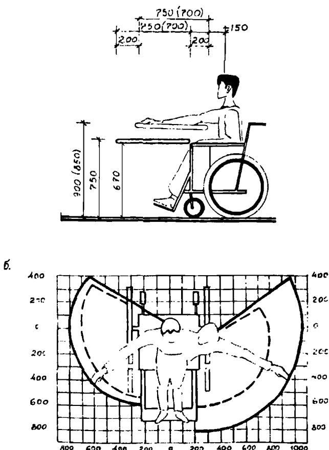
Черт. 13. Габариты трансформируемого стола (в скобках указаны размеры для женщин); оперативное поле инвалида
