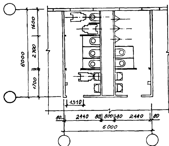
Черт. 8. Цеховая уборная с кабиной для инвалидов
