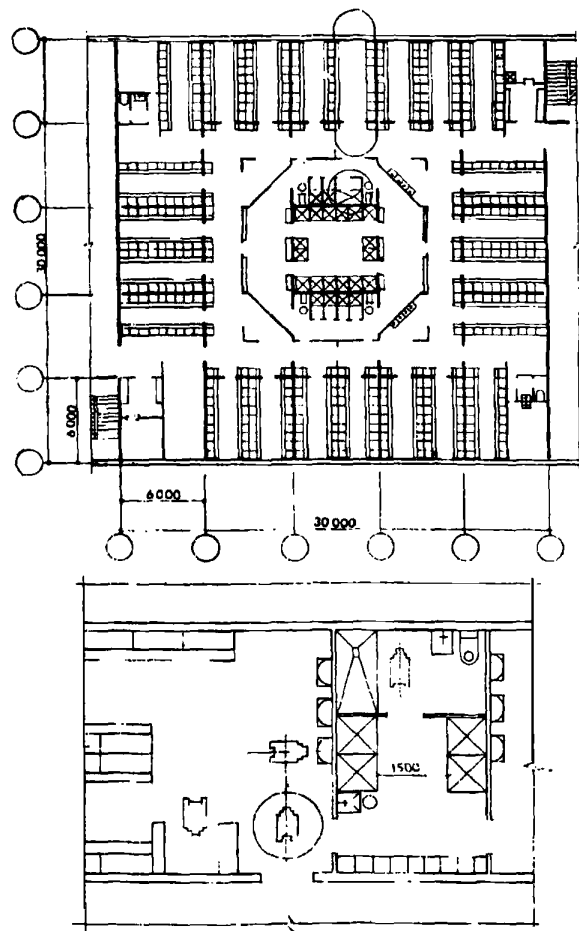
Черт. 7. Размещение гардеробной и душевой для инвалидов в общем гардеробном блоке. Индивидуальная кабина инвалида в общей душевой
