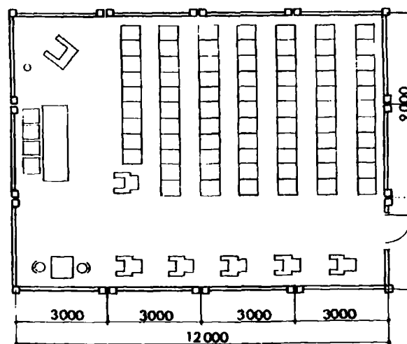
Черт. 10. Места инвалидных колясок в помещении для собраний
