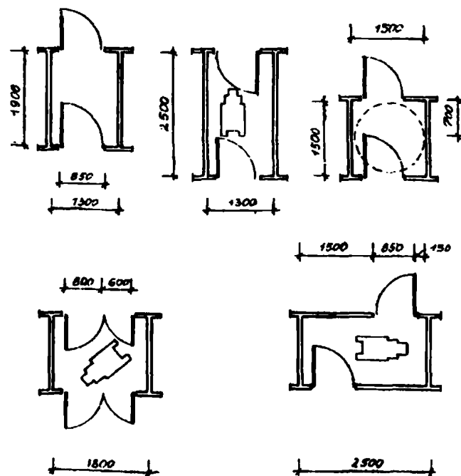
Черт. 12. Примеры устройства входных тамбуров для инвалидов
