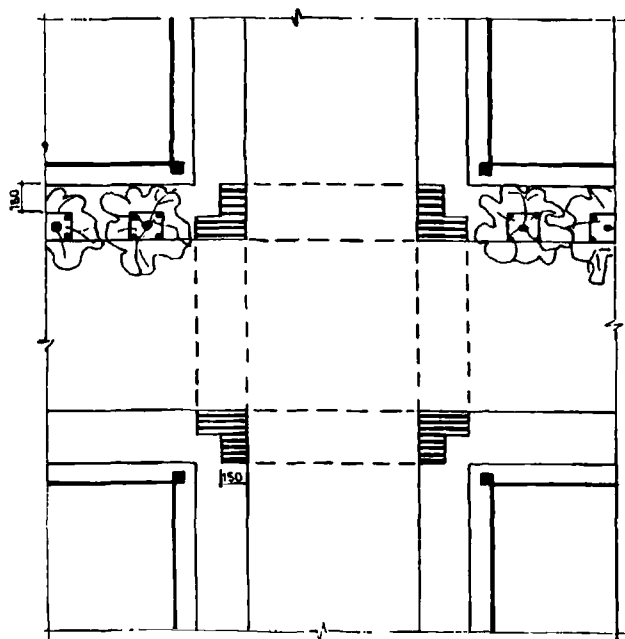
Черт. 5. Устройство внутризаводского перекрестка для слепых
