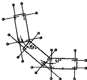
Рис. 11. Схема размещения знаков закрепления основных осей при строительстве зданий, примыкающих друг к другу под углом 45°
