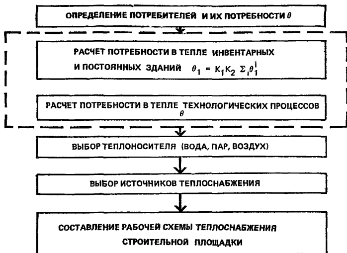
Рис. 4. Блок-схема теплоснабжения строительной площадки
