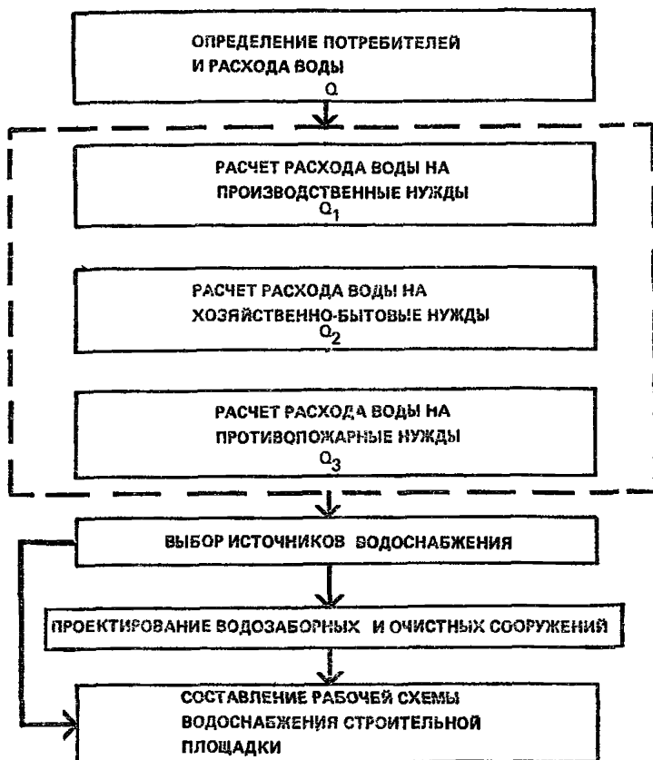
Рис. 3. Блок-схема водоснабжения строительной площадки
