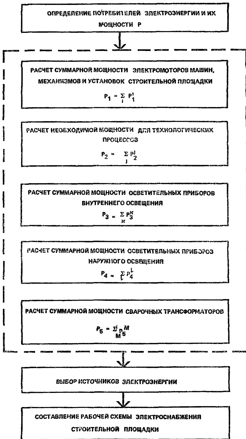
Рис. 2. Блок-схема электроснабжения строительной площадки
