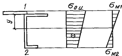
Рис. 59. Схема стрингера и эпюры нормальных напряжений
