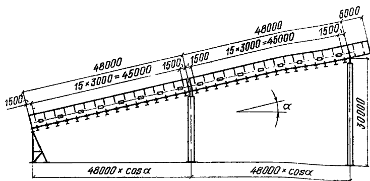
Рис. 53. Схема галереи
