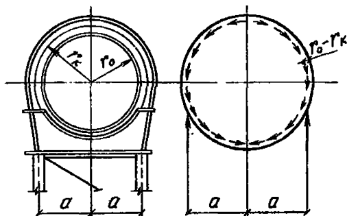
Рис. 18. Конструктивная и расчетная схема промежуточного шпангоута а -- конструктивная схема; б -- расчетная схема, 1 -- оболочка, 2 -- шпангоут, 3 -- поперечная балка-затяжка, 4 -- монорельс
