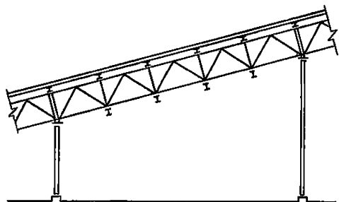
Рис. 1. Пролетное строение конвейерной галереи с несущими конструкциями из ферм с параллельными поясами
