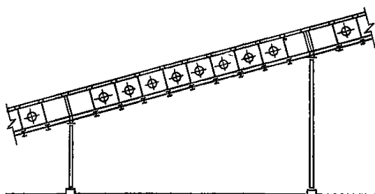
Рис. 2. Пролетное строение конвейерной галереи с несущими конструкциями из сварных двутавровых балок
