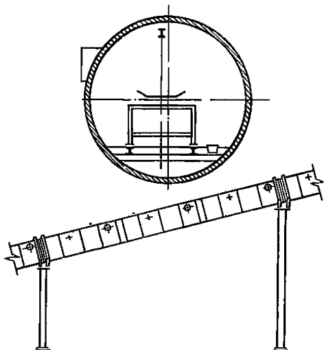
Рис. 4. Пролетное строение конвейерной галереи из круглой цилиндрической оболочки
