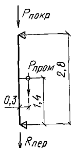
Рис. 60. Расчетная схема стойки
