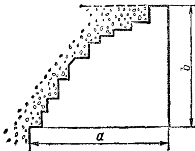
Рис. 4. Наружный карниз
