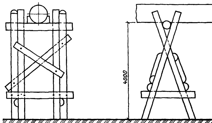
Рис. 5. Козловая опора
