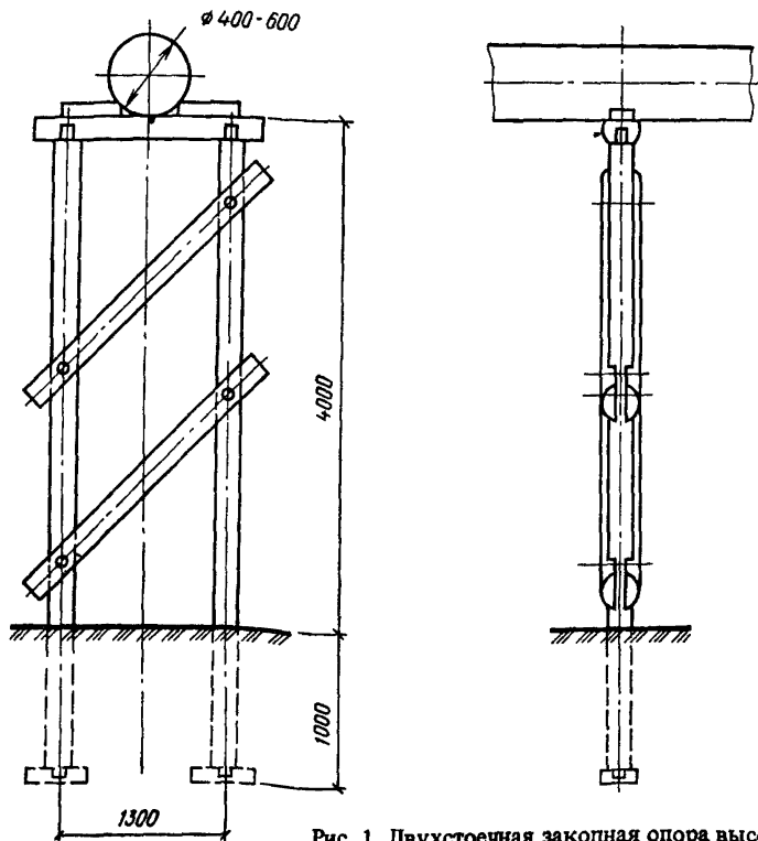
Рис. 1. Двухстоечная зацепная опора высотой 4 м
