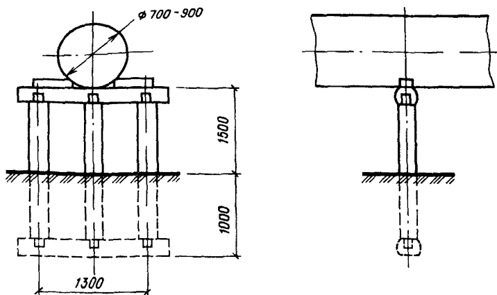
Рис. 4. Трехстоечная закопная опора высотой 1,5 м
