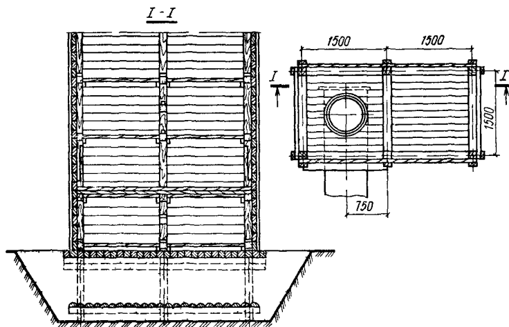
Рис. 8. Двухсекционный деревянный водосбросной колодец с трубчатым стояком высотой св. 6 м.
