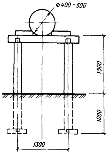
Рис. 2. Двухстоечная закопная опора высотой 1,5 м
