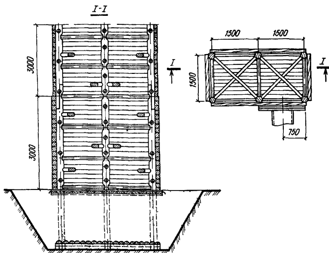
Рис. 9. Двухсекционный деревянный водосбросной колодец высотой до 6 м
