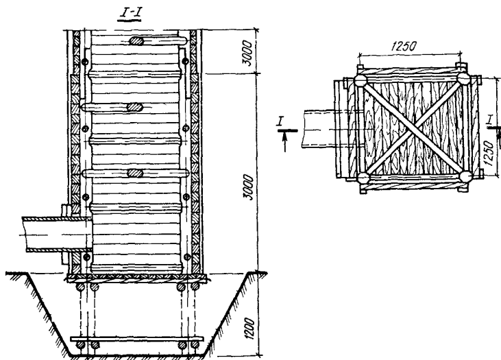
Рис. 7. Односекционный деревянный водосбросной колодец высотой до 6 м
