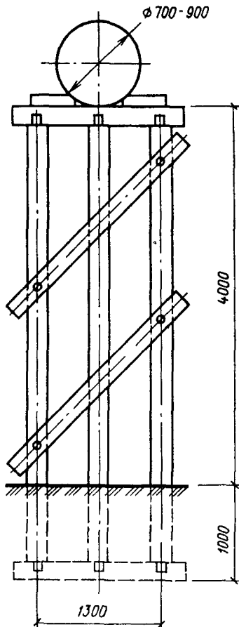
Рис. 3. Трехстоечная закопная опора высотой 4 м
