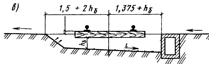
Рис. 1. Поперечные профили балластной призмы
