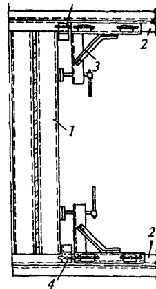
Рис. 9. Схема поэлементной сборки ограждения из профильного стекла
