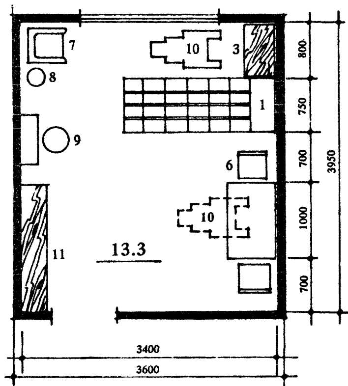
Рис. 1. Планировочная схема одноместной спальни комнаты. (Вариант при шаге 3,6 м). Экспликация оборудования: 1 — кровать 190x70, 2 — диван 200x75, 3 — тумбочка 40x80, 4 — тумбочка 40x40, 5 — стол 60x100, 6 — стул 40x40, 7 — кресло 50x50, 8 — торшер, 9 — банкетка, 10 — инвалидная коляска, 11 — комбинированный шкаф
