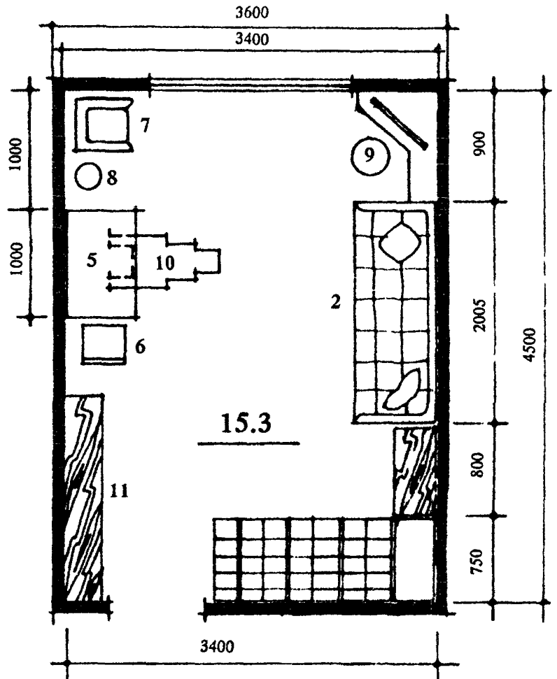
Рис 5. Планировочная схема спальни на 2 места. (Вариант при шаге 3,6 м). Эхспликаци. оборудования см. рис. 1.
