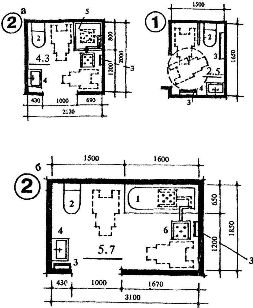
Рис. 8. Планировочные схемы санитарных узлов. Вариант 1 — Уборная с умывальником. Вариант 2 — Санитарный узел при спальном комнате (а — вариант с душем, б — вариант с ванной). Эクスпликация оборудования: 1. ванна 65x160, 2. унитаз 40x60, 3. вешалка для полотенец, 4. умывальник 60x40, 5. душевой поддон 80x80, 6. поворотное кресло.
