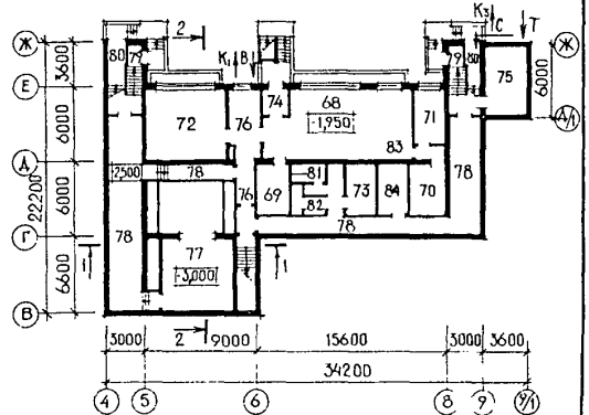
ПЛАН ЦОКОЛЬНОГО ЭТАЖА И ПОДВАЛА
