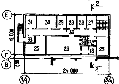
ПЛАН НА ОТМ. 3,000
