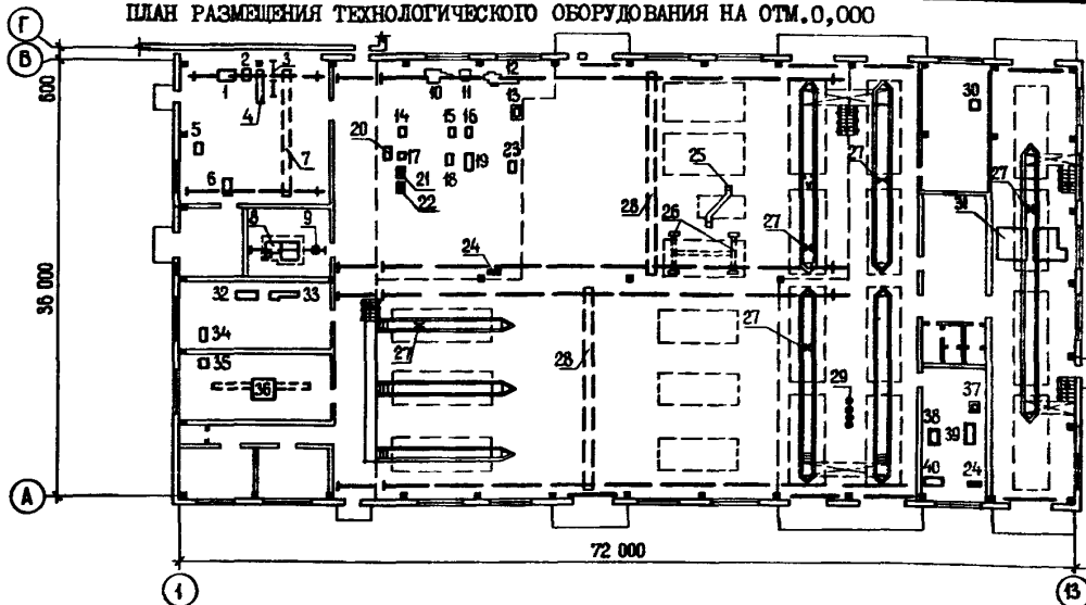
ПЛАН РАЗМЕЩЕНИЯ ТЕХНОЛОГИЧЕСКОГО ОБОРУДОВАНИЯ НА ОТМ. 0,000
