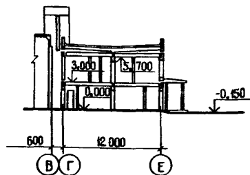
РАЗРЕЗ 2-2
