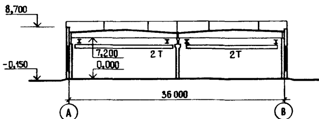
РАЗРЕЗ I-I
