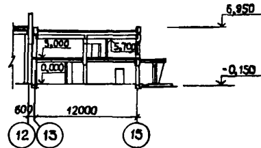
РАЗРЕЗ 2-2
