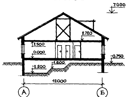
РАЗРЕЗ I-I
