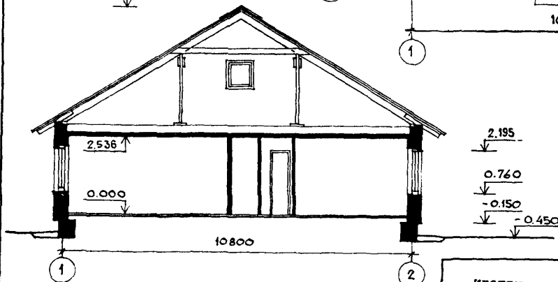
РАЗРЕЗ I-I
