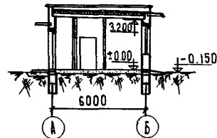
РАЗРЕЗ I-I
