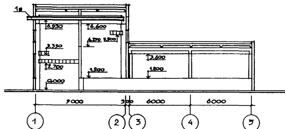
РАЗРЕЗ I-I
