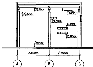
РАЗРЕЗ 2-2
