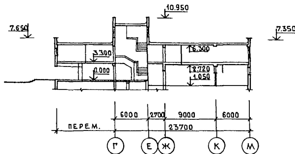
РАЗРЕЗ I-I
