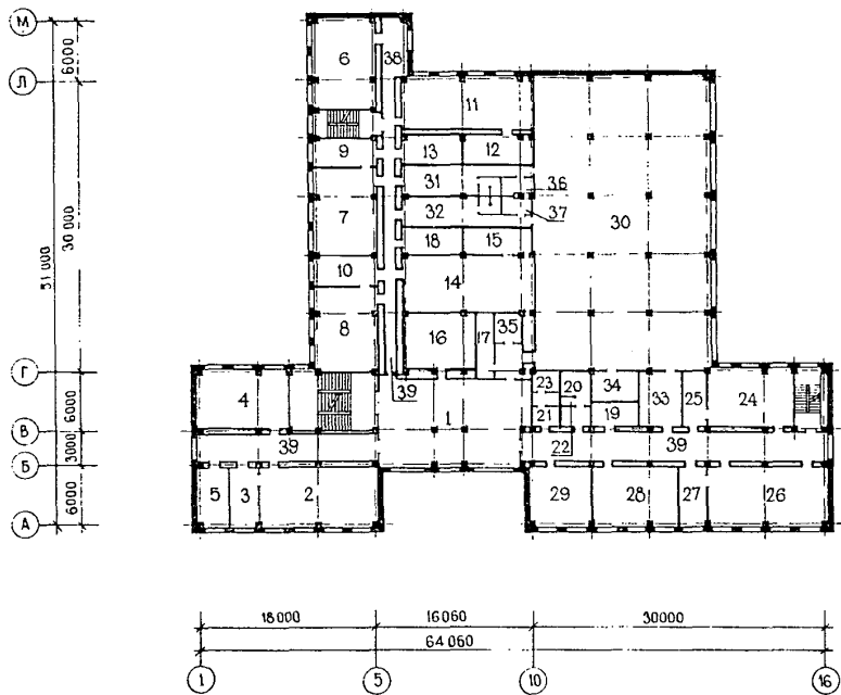
ПЛАН 2 ЭТАЖА
