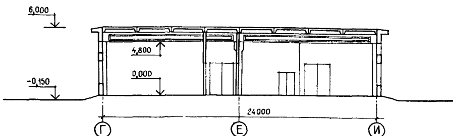
РАЗРЕЗ I-I
