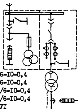
СХЕМЫ ЭЛЕКТРИЧЕСКИХ СОЕДИНЕНИЙ
