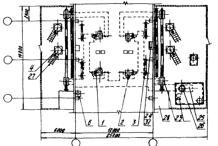
ВАРИАНТ 3 ПЛАН НА ОТМ. 0,000
