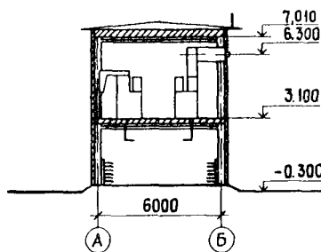
РАЗРЕЗ А-А
