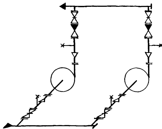
двух насосов
