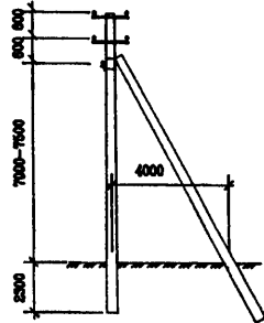
Угловые анкерные
