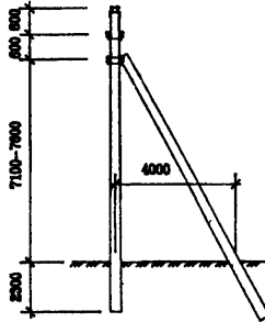
Концевые (анкерные)
