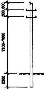
Промежуточные
