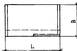
Рис. 3 Площадки верхние
