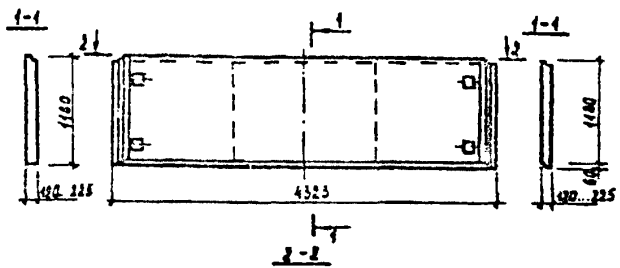
Полигональный блок рядовой
